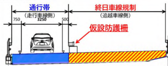
追越車線規制概略断面図
