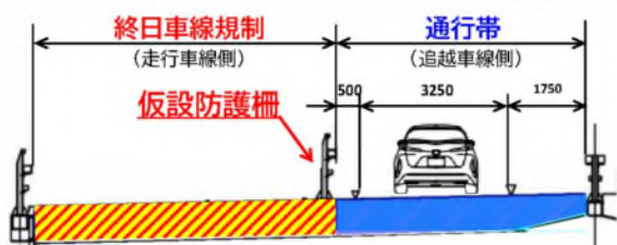
走行車線規制概略断面図
